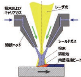
図1 レーザクラディングの概念図
