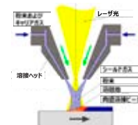
図1 レーザクラディングの概念図
